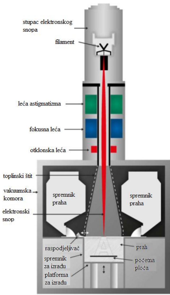
Slika 3.11. Dijelovi EBM 3D pisaača
