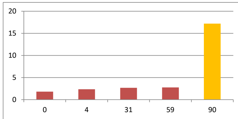
Graf 4.1.4. Sadržaj β-kriptoksantina u sjenaži i paši (µg/g suhe tvari)
