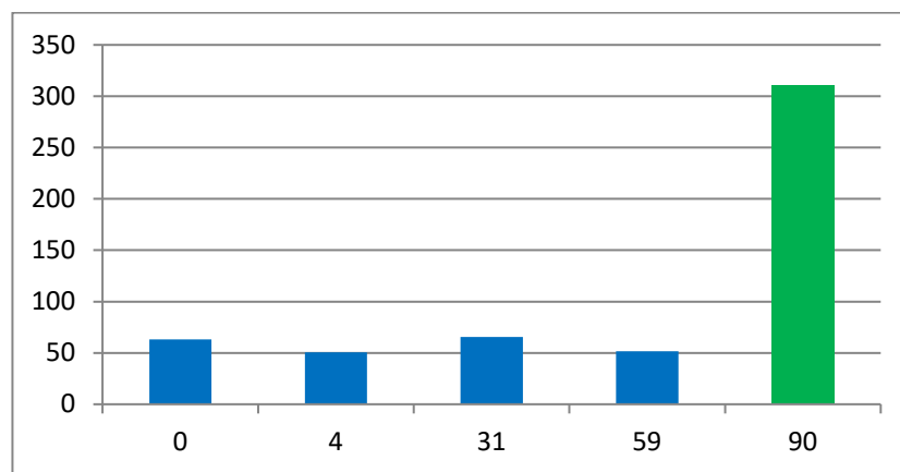
Graf 4.1.5. Sadržaj β-karotena u sjenaži i paši (µg/g suhe tvari)
