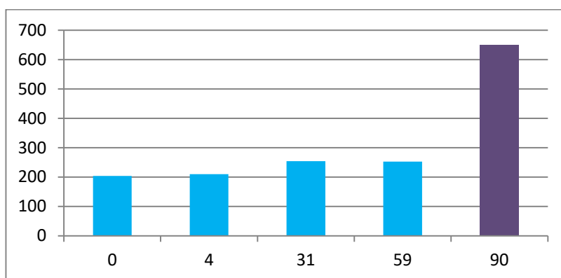
Graf 4.1.3. Sadržaj luteina u sjenaži i paši ( \mu\text{g/g} ST)
