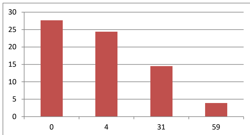
Graf 4.1.2. Sadržaj \beta -karotena u sijenu ( \mu\text{g/g} )
