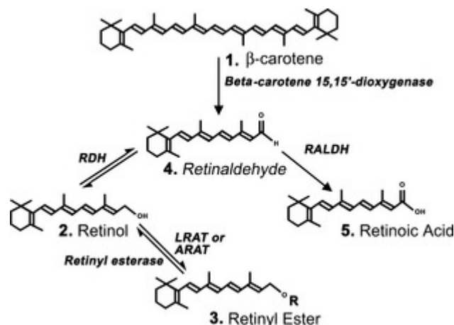
Slika 2.4.1. Kemijska struktura \beta karotena i tri oblika retinola
