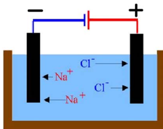
Slika 9: Konduktometrijsko mjerenje
