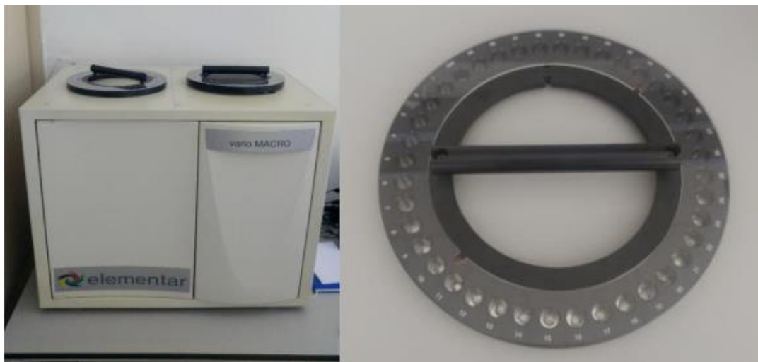
Slika 4.3. Prikaz CHNS analizatora s autosamplernom
