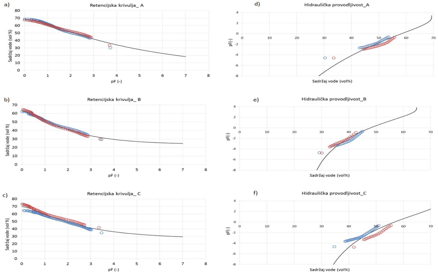
Slika 14. Retencijske i hidrauličke krivulje dobivene pomoću HYPROP-FIT programa koristeći podatke evapotranspiracijske metode dobivene HYPROP uređajem; slike a),b),c) prikazuju retencijske krivulje za jako opožareno, opožareno i kontrolno tlo dok slike d),f),e) prikazuju krivulje provodljivosti za jako opožareno, opožareno i kontrolno tlo. Crne linije predstavljaju krivulje projicirane na temelju izmjerenih vrijednosti relativne količine vode u tlu i vodnog potencijala tla a temelje se na VGM modelu
