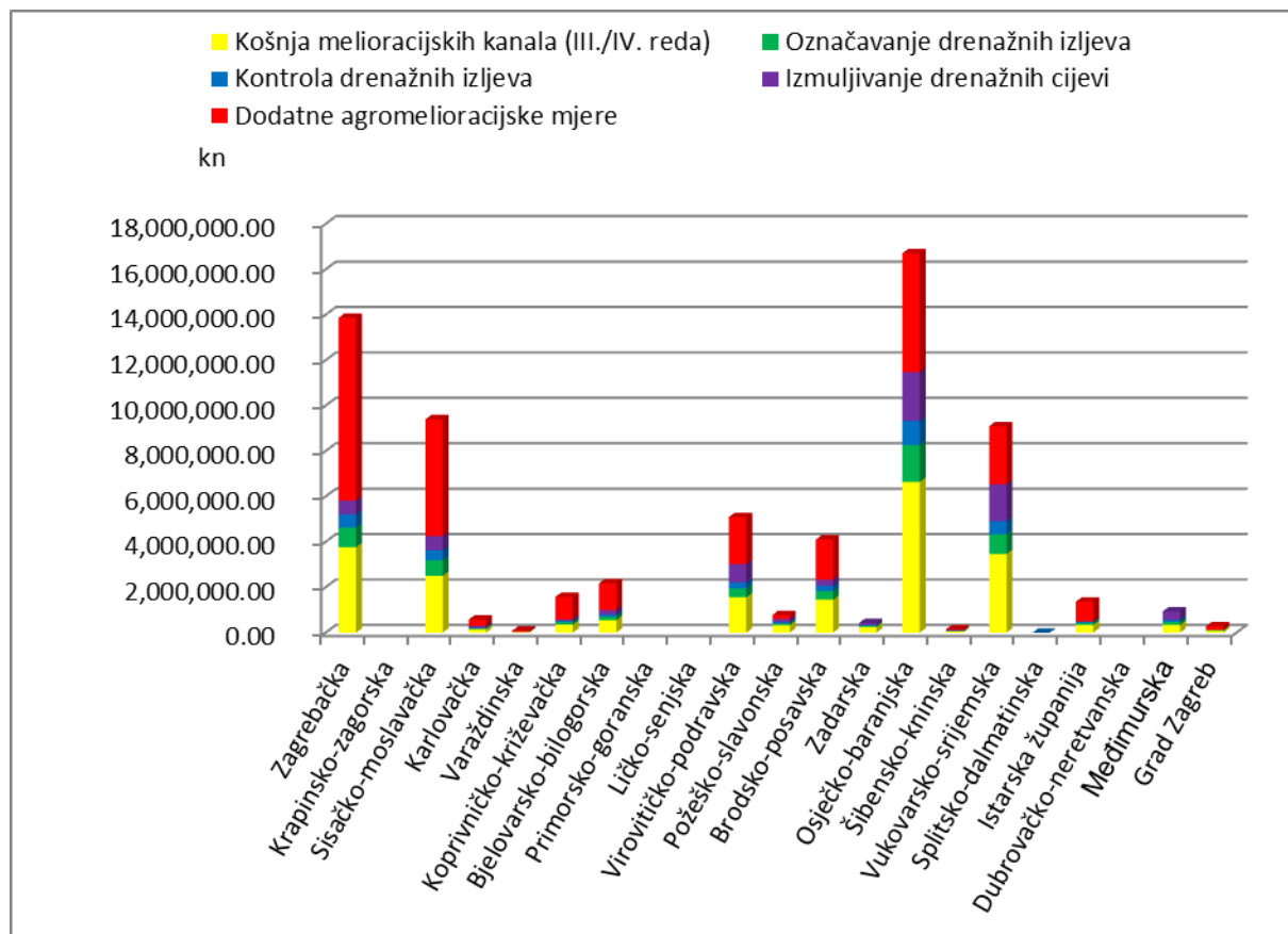
Grafikon 16. Prijedlog mjera za redovito održavanje obnovljenih kombiniranih sustava površinske i podzemne odvodnje po županijama u RH
