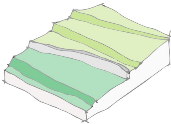
Slika 3.39. Terasirana polja
