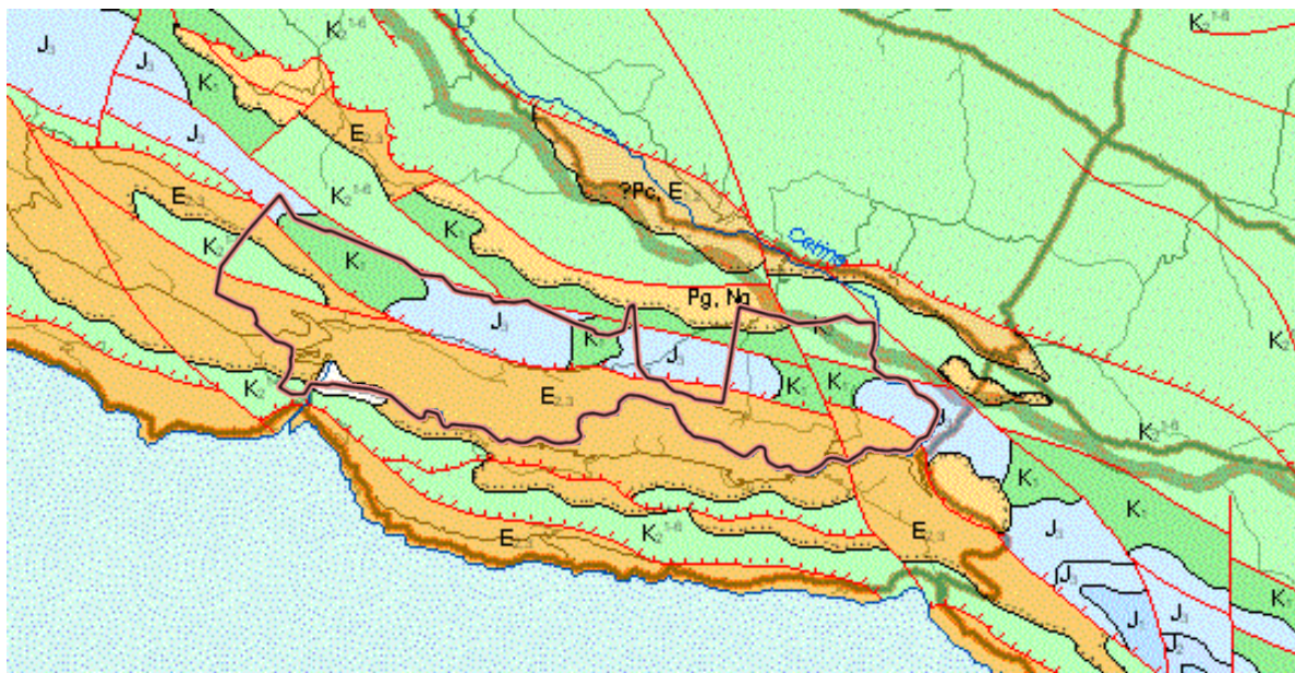
Slika 4.: Geološka karta Hrvatske 1:300.000, Omiško zaobalje (izvor: http://webgis.hgi-cgs.hr/gk300/default.aspx )
