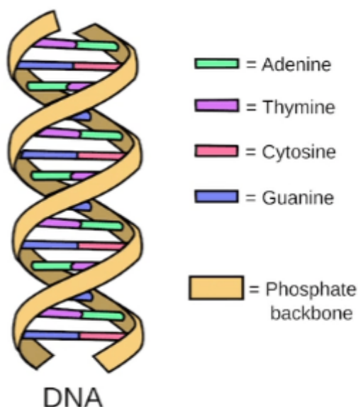
Slika 3. Struktura DNA
