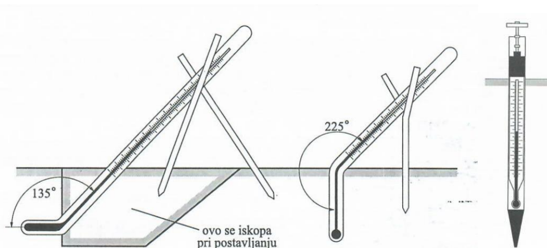
Slika 2.2.1. Koljenasti geotermometar svinut pod kutom 135°C i 225°C i oklopni geotermometar
