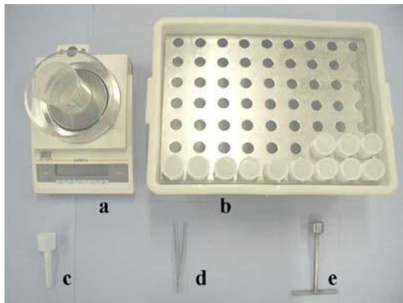
Slika 7. Alati za određivanje EZ metode: a) Vaga (10 mg), b) držač za kontejnere, c) kontejner, d) pinceta, e) sonda (Ø25mmx25mm). (izvor: Danish Meat Research Institute, 2010)
