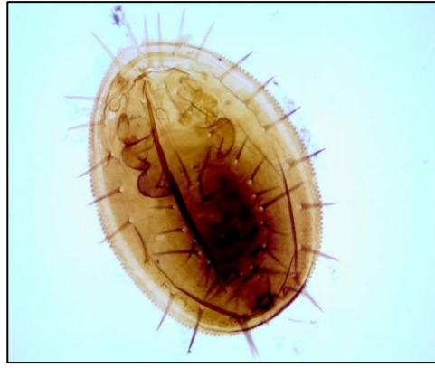
Slika 41. Aleurocanthus spiniferus , mikroskopski preparat puparija (povećanje 100x)
