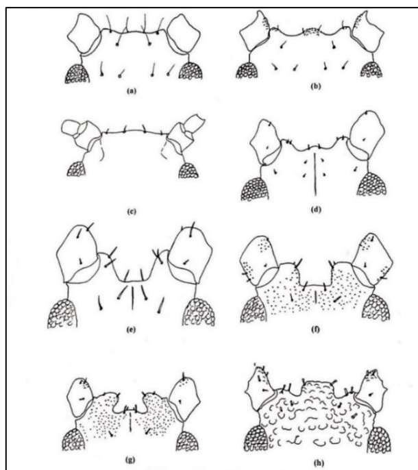
Slika 17. Leđna strana glave različitih vrsta iz potporodice Aphidinae koja pokazuje razlike u obliku glave i razvijenost antenskih tuberkula (izvor: Blackman i Eastop, 2000)
