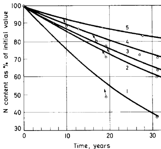
Slika 2.4.1. Utjecaj kultivacije na karakter transformacije organske tvari. 1. kontinuirani kukuruz; 2. kontinuirana pšenica; 3. Kontinuirana zob; 4. Petoredni plodored: kukuruz, zob, pšenica, djetelina i mačji repak; 5. Plodored u tri reda: kukuruz, pšenica i djetelina.
