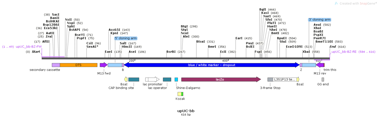
Slika 14. Amplicinski fragment za marker za plavo-bijelu selekciju iz pBacBoneBZ_ann plazmida (upUC-bb)
