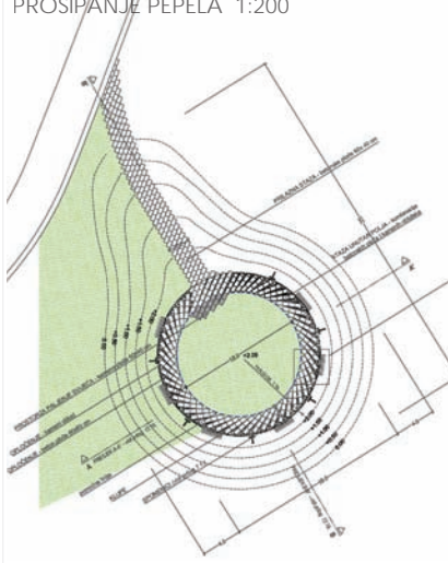
PROSIPANJE PEPELA 1:200
