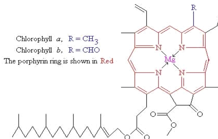
Slika 2.3. molekula klorofila
