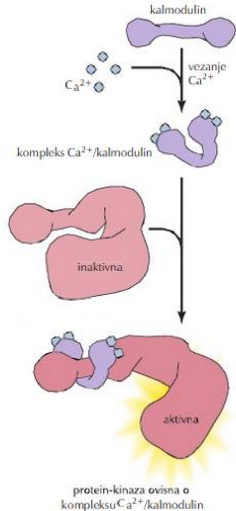
Slika 1. Kalmodulin ima oblik bučice s četiri vezna mjesta za kalcij
