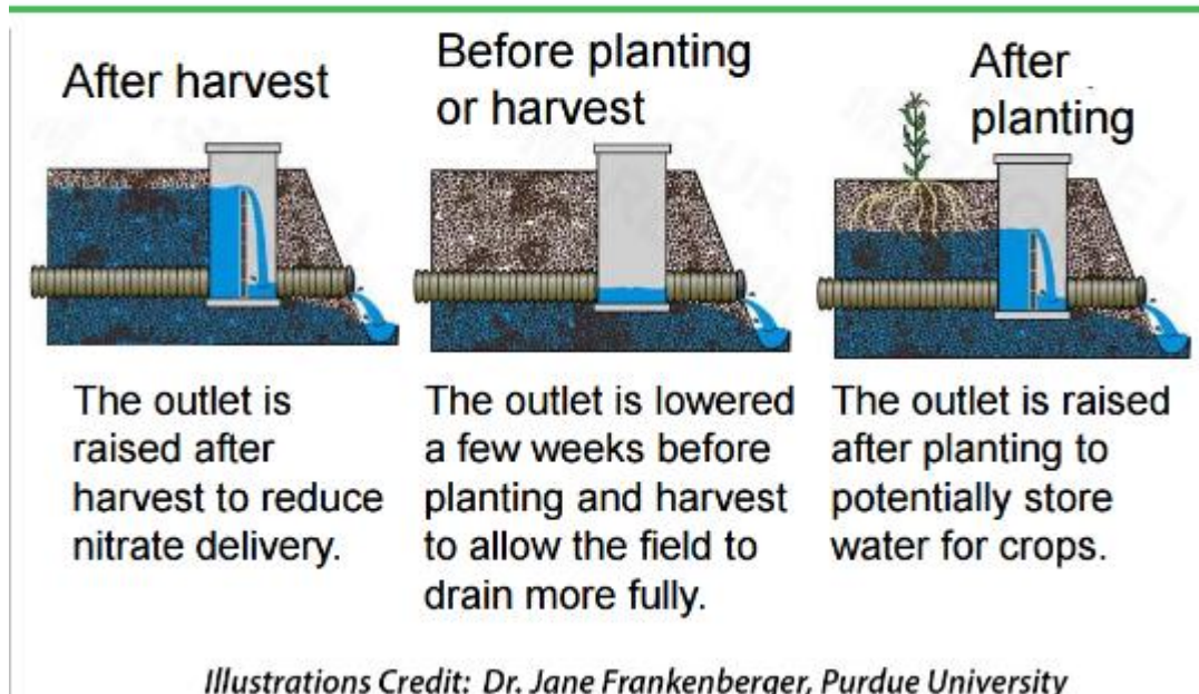
Slika 12. Upravljanje razinom drenažne vode Izvor: Frankenberger
