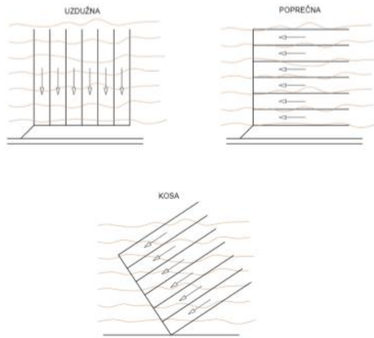
Slika 5. Tipovi drenaže Izvor: Petošić
